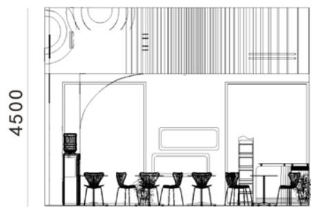
6000 正面图
