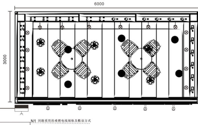
电气平面图 (供参考)
