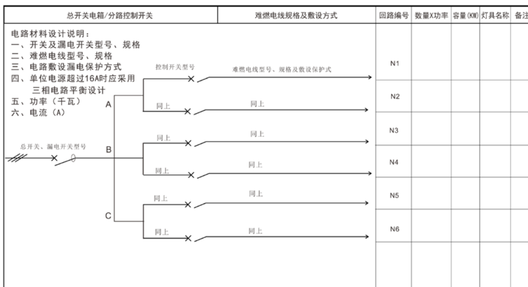
特装摊位配电系统图 (供参考)
